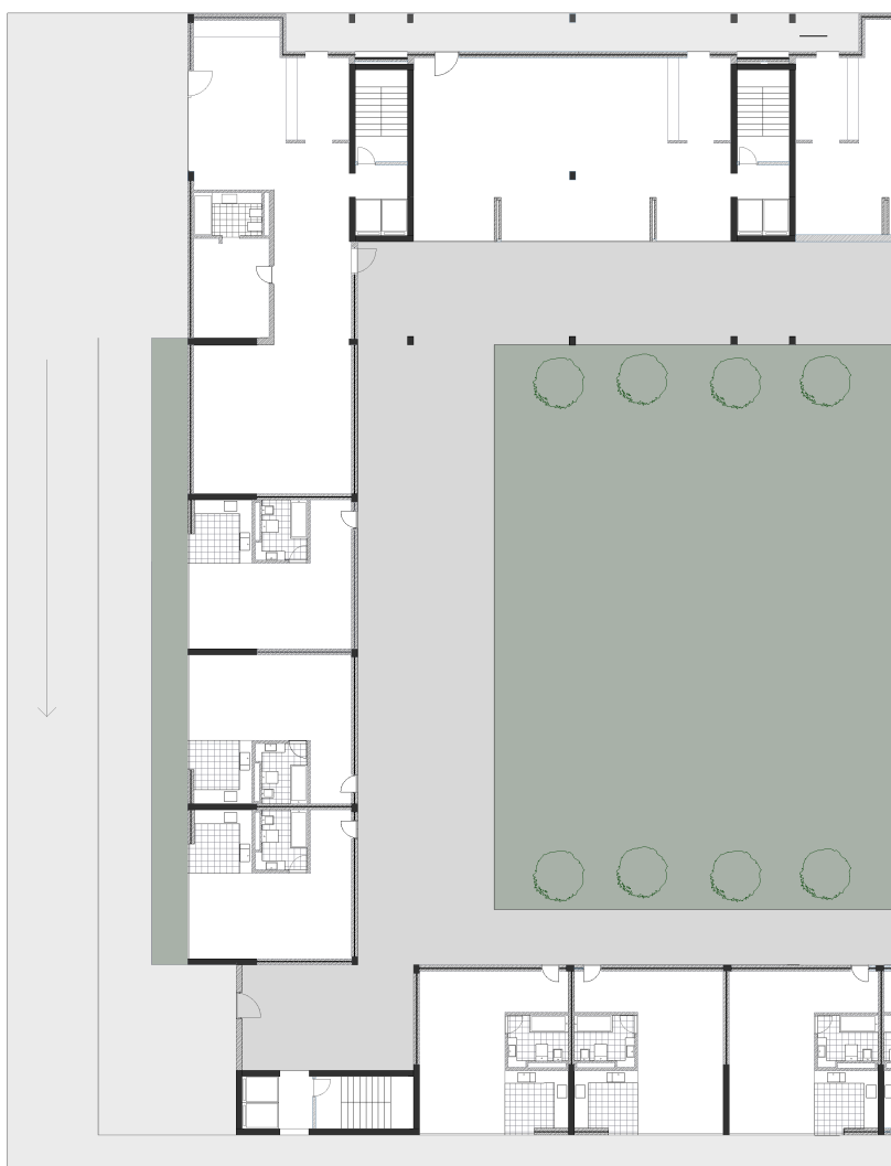
01 planta do rés-do-chão — comércio, habitação T0 e logradouro (desenho original 1:100, reduzido)
